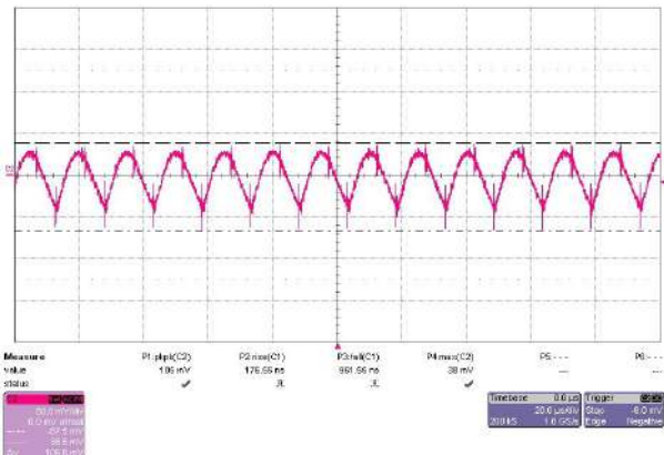
FS15-15 106.0mVpp
