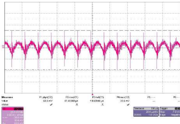
FS15-12 68.6mVpp
