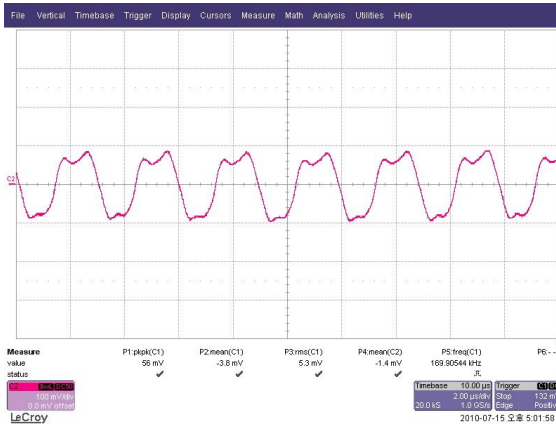
[Fig.5] Input reflect ripple current (100mA/div)
